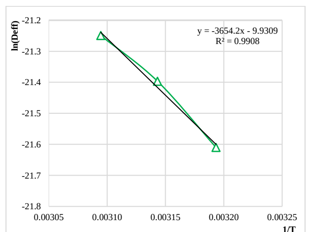
Hình 10. Đồ thị quan hệ E_a và D_{eff} tại P=160W
