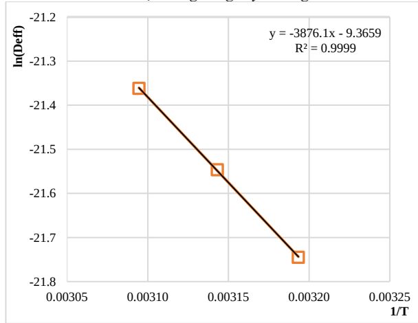
Hình 6. Đồ thị quan hệ E_a và D_{eff} tại P=80W
