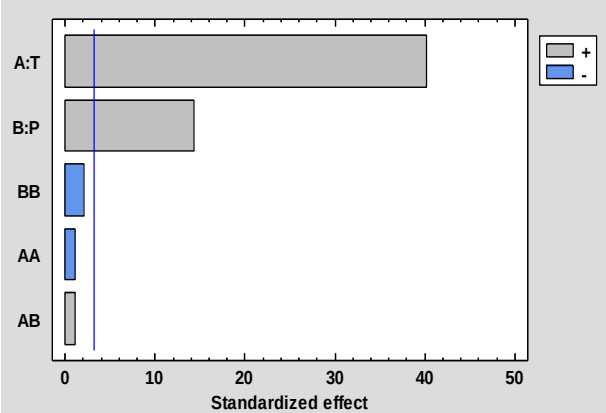
Hình 3. Ảnh hưởng các hệ số hồi quy đến hệ số khuếch tán ẩm D_{eff}
