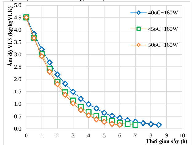
Hình 9. Đồ thị đường cong sấy ở công suất 160W
