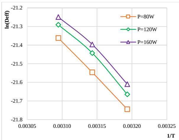
Hình 10. Đồ thị quan hệ E_a và D_{eff} các mức công suất sóng siêu âm khác nhau
