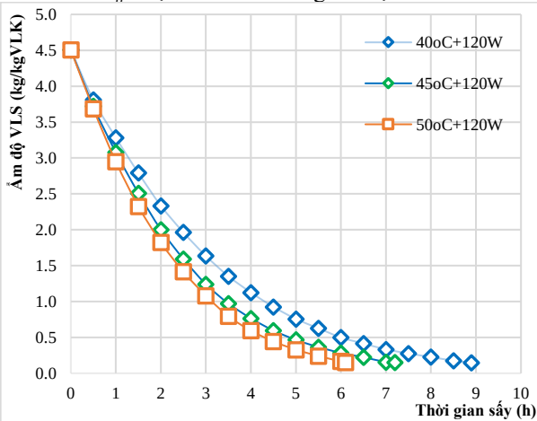
Hình 7. Đồ thị đường cong sấy ở công suất 120W
