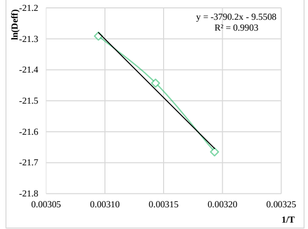
Hình 8. Đồ thị quan hệ E_a và D_{eff} tại P=120W
