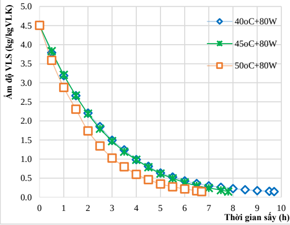
Hình 5. Đồ thị đường cong sấy ở công suất 80W
