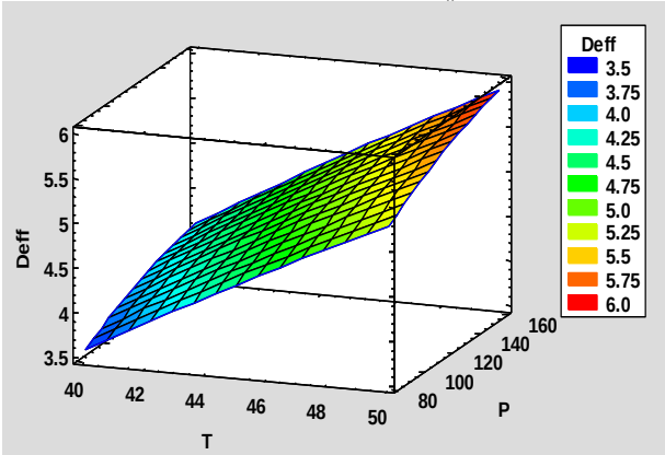
Hình 4. Ảnh hưởng nhiệt độ, công suất đến hệ số khuếch tán ẩm D_{eff}
